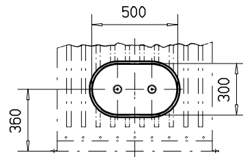
③ Beobachtungsdeckel Inspection cover Porte de visite
